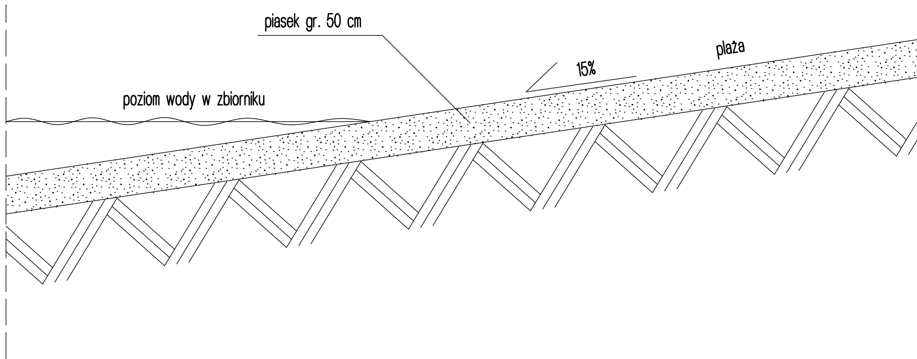
PRZEKRÓJ PRZEZ PLAŻĘ PRZY ZBIORNIKU WODNYM 1:50
