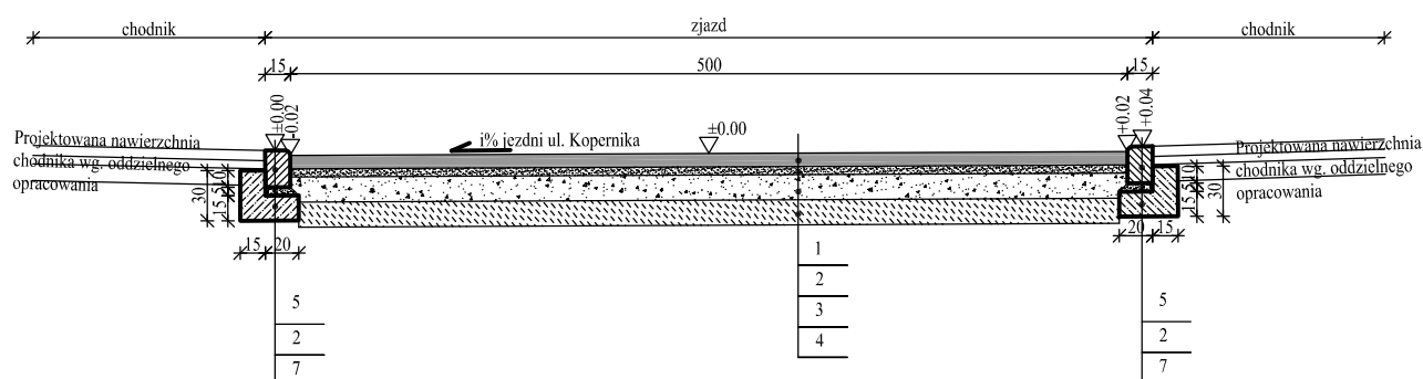
Przekrój normalno - konstrukcyjny II-II - chodnik, zjazd
