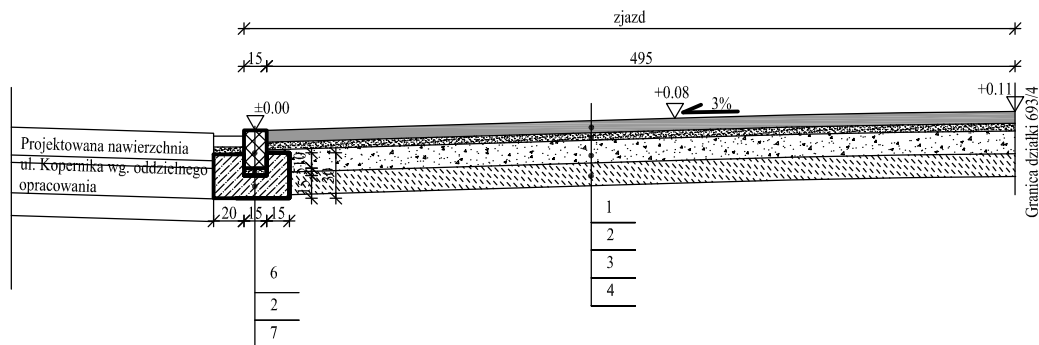
Przekrój normalno - konstrukcyjny II-II - chodnik, zjazd
